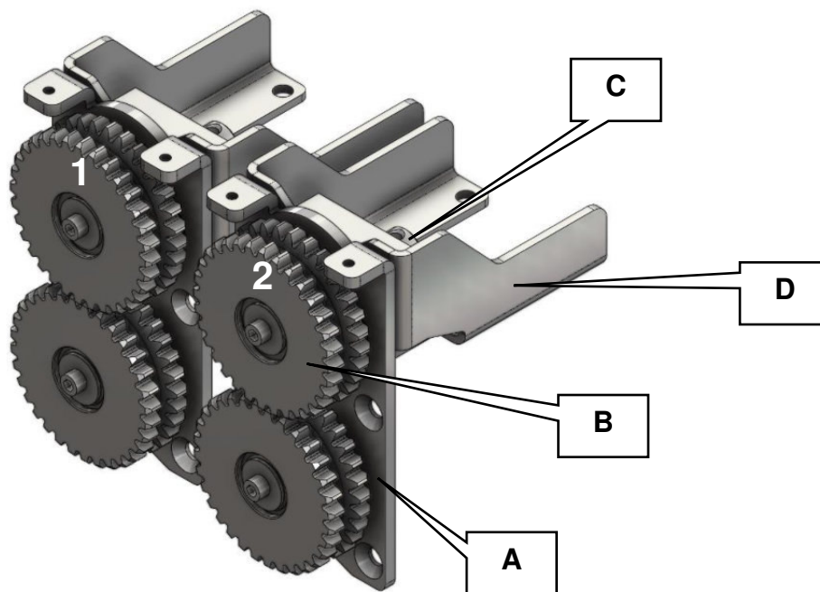
Le due trasmissioni laterali
